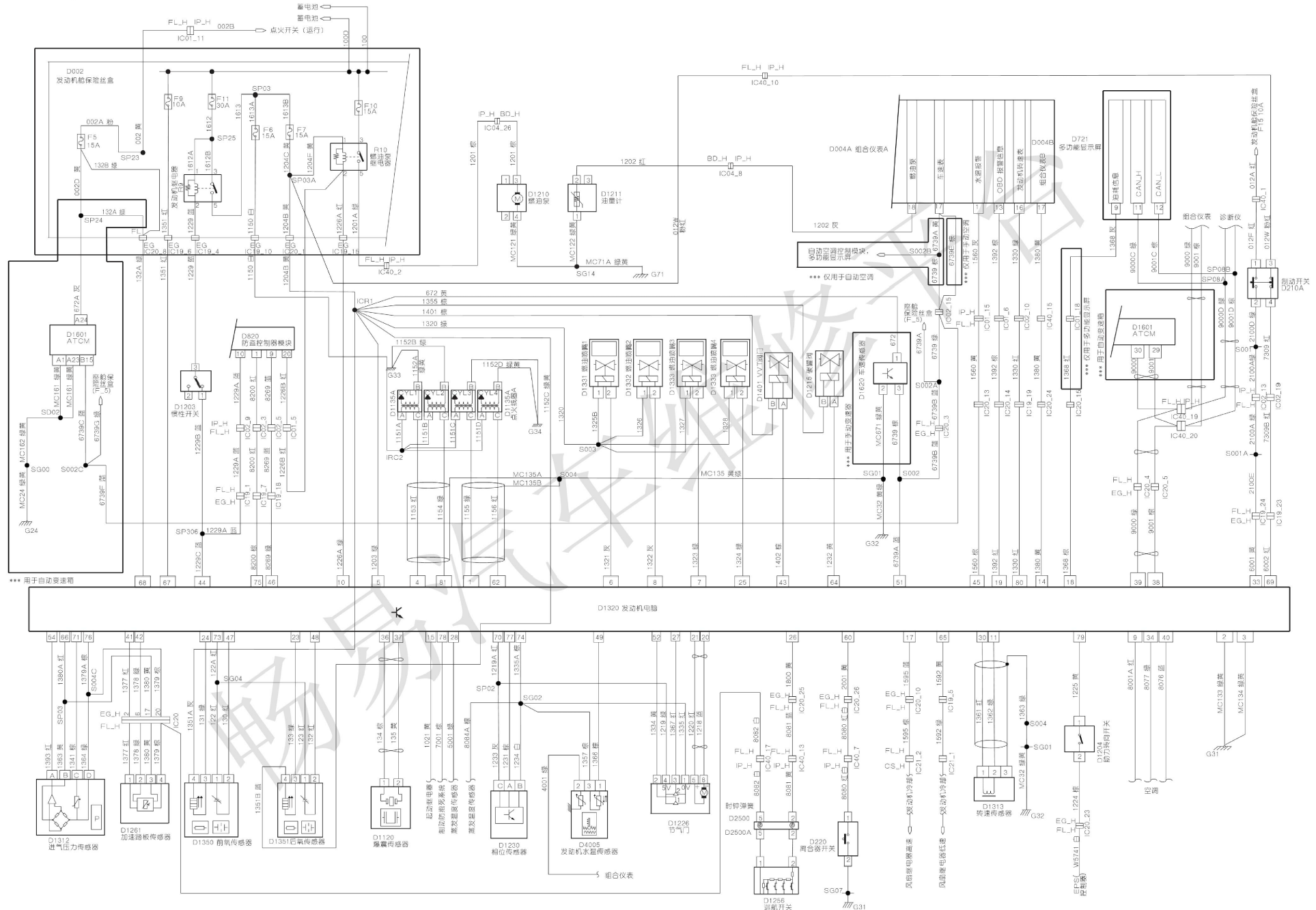
发动机控制电器原理图
